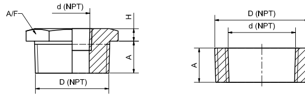
Dimensions Table
