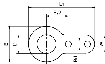
Paddle Spacer
