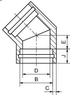
Dimensions Table 45°
