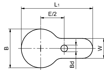
Paddle Blank
